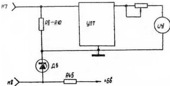
Черт.6. Упрощенная схема омметра.
