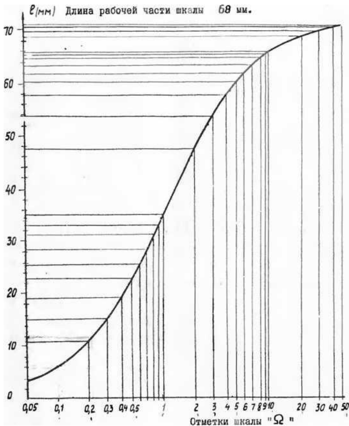
График соответствия отметок шкалы " \Omega " прибора В7-15 длине шкалы в миллиметрах. (График усредненный для шкал О, Б, В, Г и Д микроамперметра М1690А).
