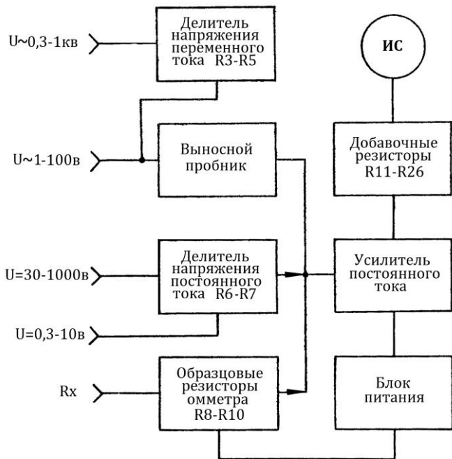
Черт. 4. Блок-схема прибора.
