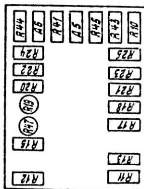
Плата № 7.102.004
